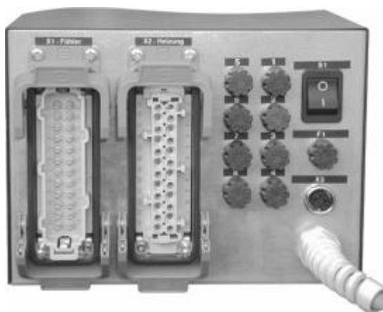
MCSe8 (Beispiel mit 24-pol. Steckern)
