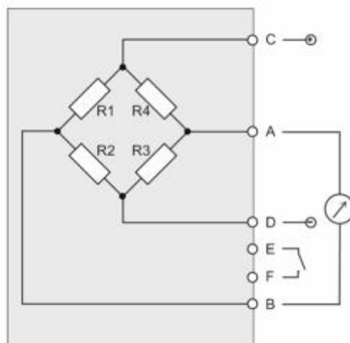
Ersatzschaltbild des DMS-Druckaufnehmers (Wheatstone-Brücke)
